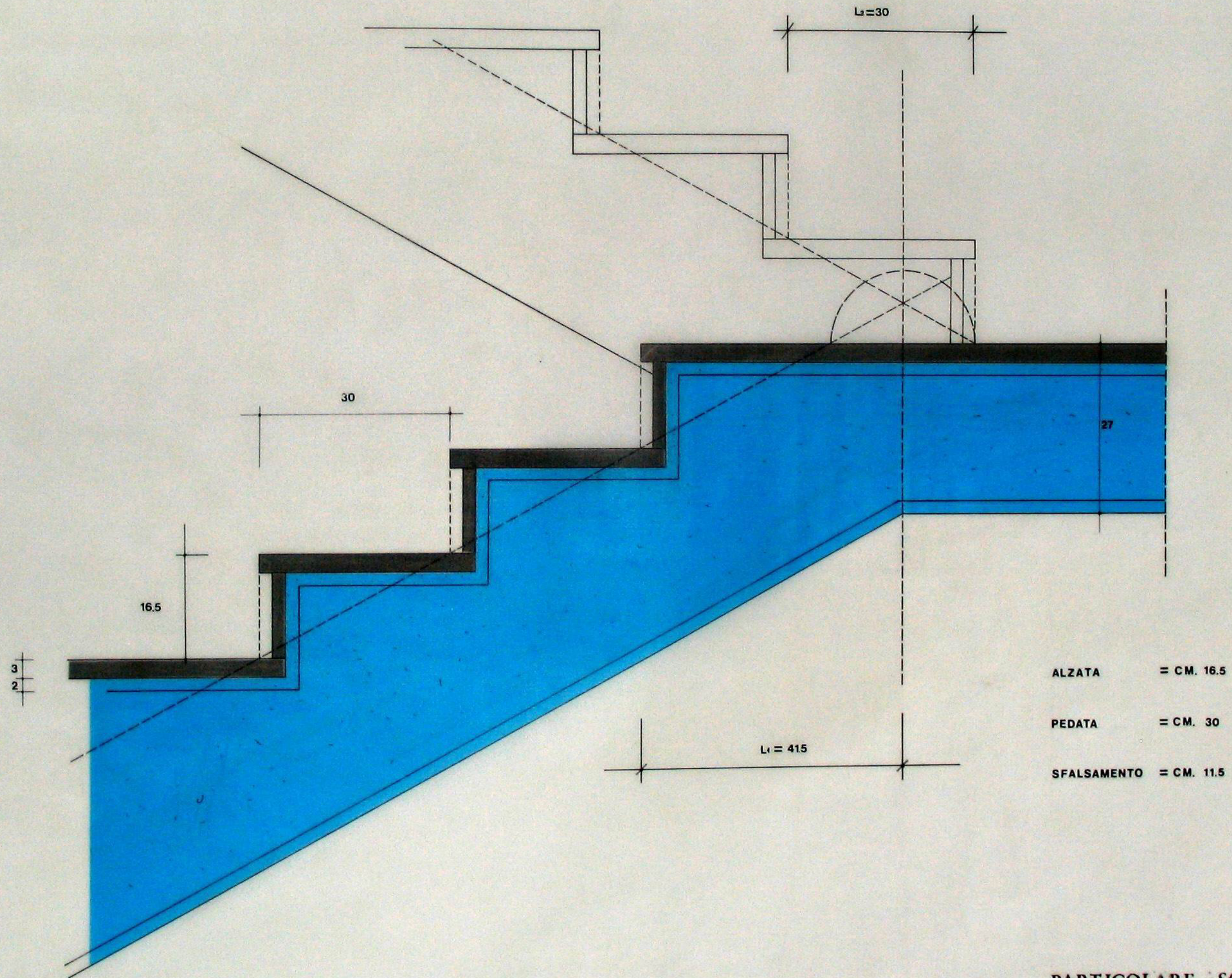
PARTICOLARE SCALA 1:5
